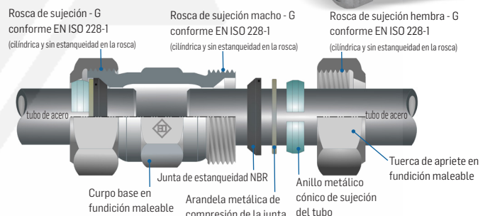
Ejemplo 6 Junta rápida macho marca EO, ref.º 746
