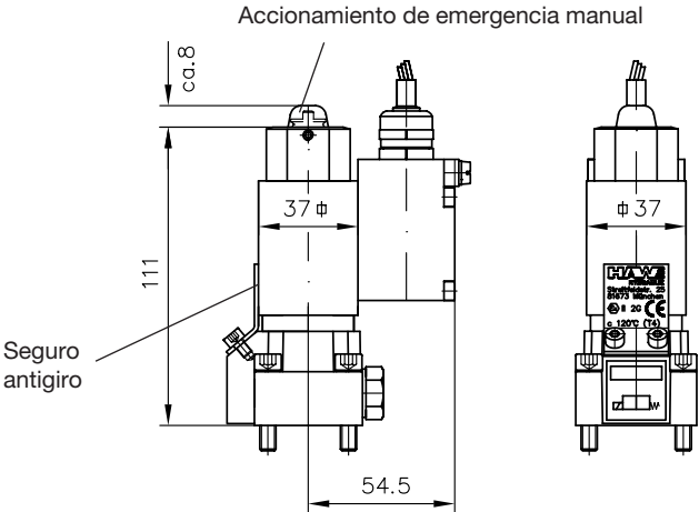
Tamaño 1 bobina antideflagrante
